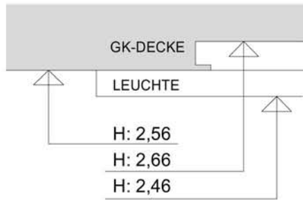
HÖHENSCHHEMA DECKE
